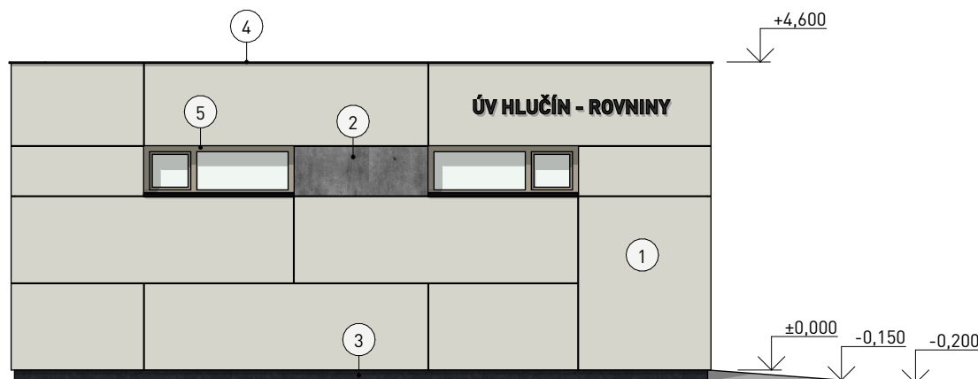
POHLED SEVEROZÁPADNÍ
