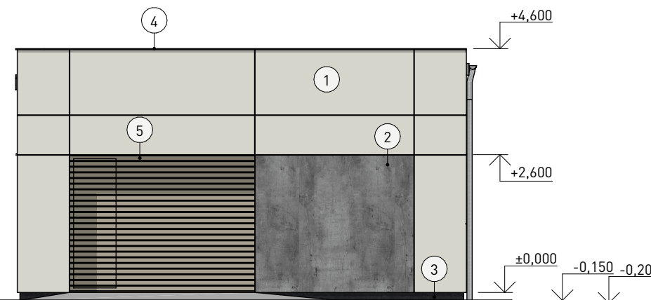
POHLED JIHOZÁPADNÍ
